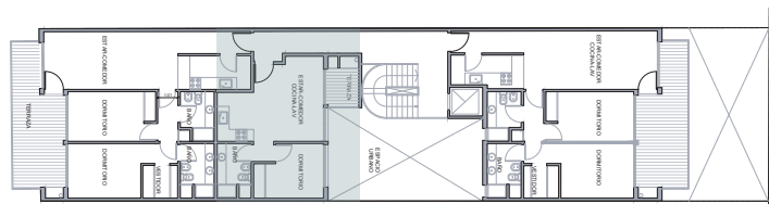
PRIMER PISO
