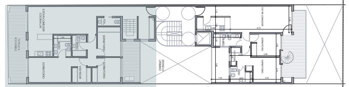
SEGUNDO PISO
