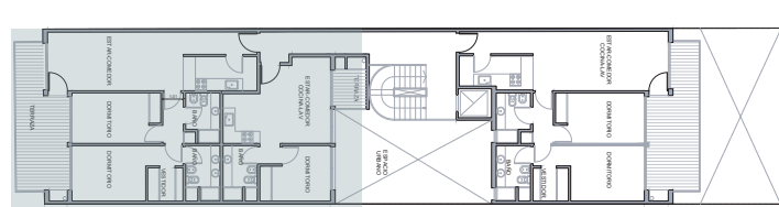
TERCER PISO
