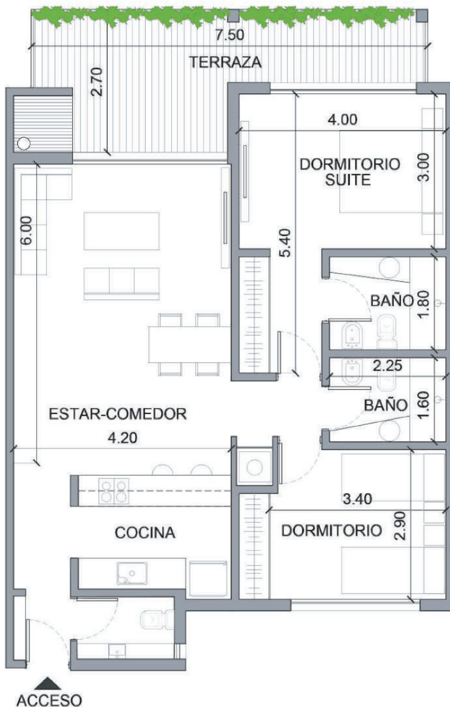
TERCER PISO
