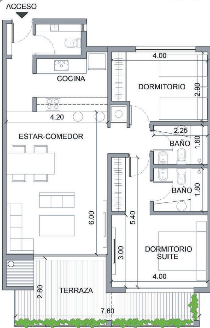
SEGUNDO PISO
