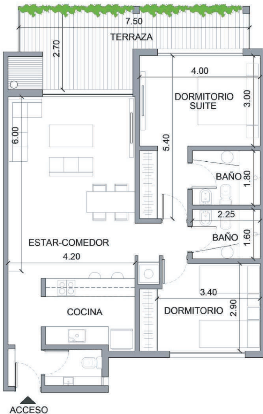
SEGUNDO PISO
